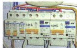
Рис. 91. Современный квартирный щиток с предохранителями
