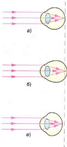
Рис. 165. Недостатки зрения
