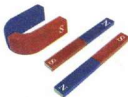
Рис. 108. Постоянные магниты
