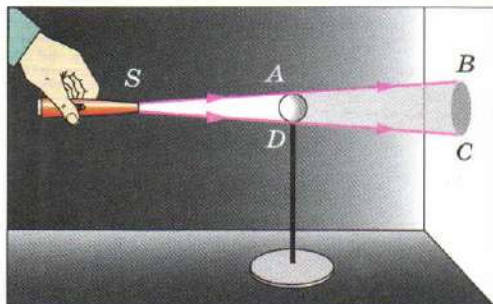
Рис. 123. Получение тени
