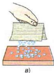
Рис. 30. Электризация трением
