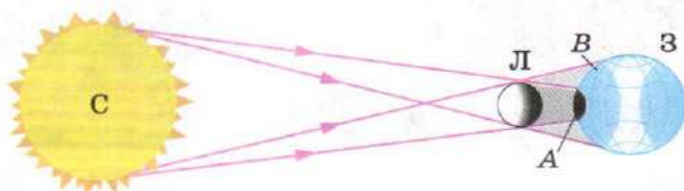
Рис. 126. Солнечное затмение
