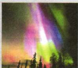
Северное сияние
