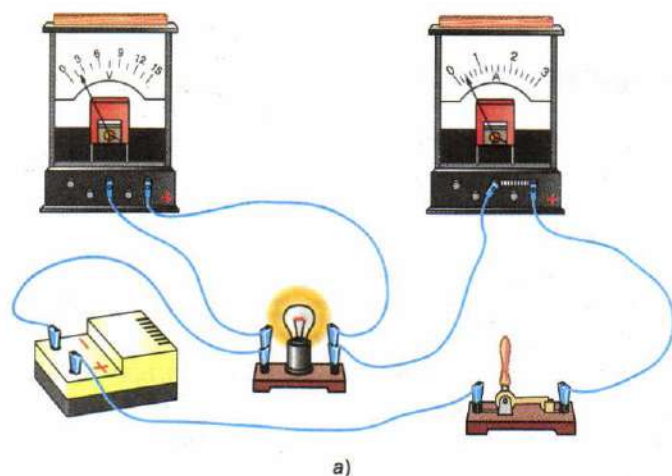
Рис. 66. Подключение вольтметра и амперметра в цепь
